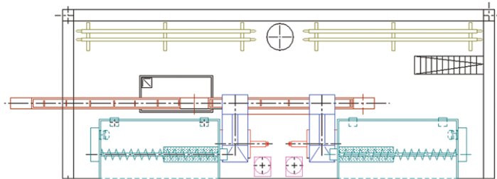
Технологическая схема /план/ стандартной приемной линии Technological line /space plan/ of standart receiving line
